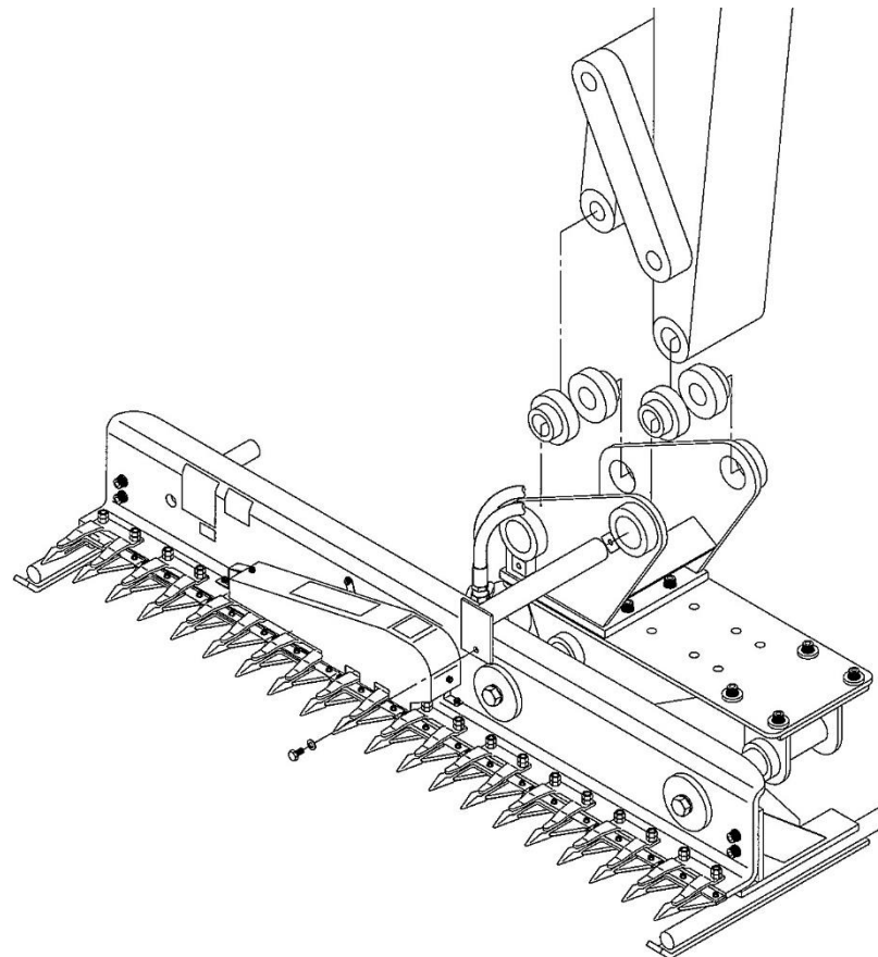
図4. 小型油圧ショベルへの取り付け方法
