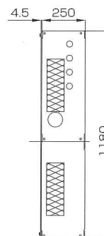
外観図は、ABS-212 ABS-210S/210/206S/206も同寸法
