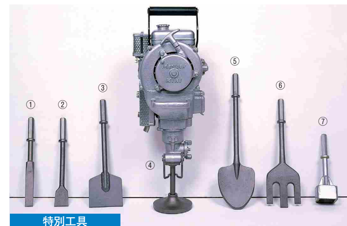
①チゼル ②カッター ③アスファルトカッター ④タンピングランマー ⑤ショベル ⑥リッパー ⑦バイルハンマー
