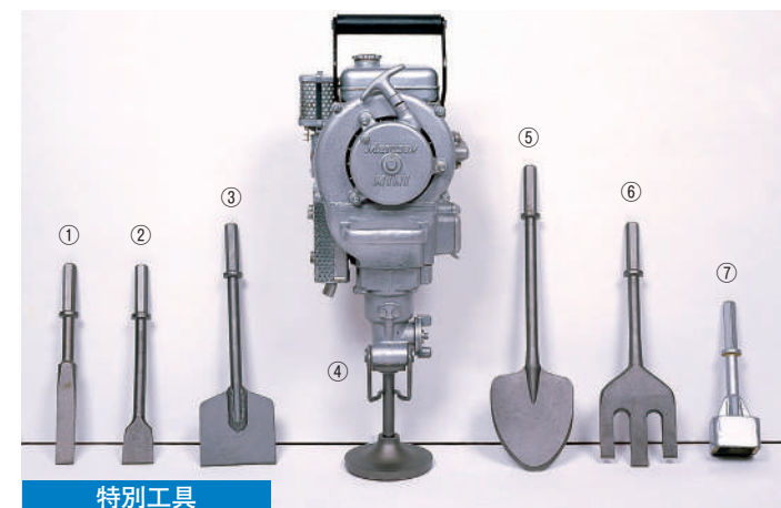
①チゼル ②カッター ③アスファルトカッター ④タンピングランマー ⑤ショベル ⑥リッパー ⑦パイルハンマー
