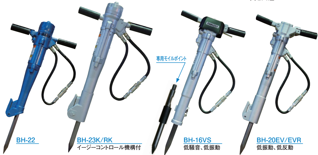
油圧ショベル、クレーン車などの建設車両からも油圧を取り出して、各種油圧ハンドブレーカが使用可能！
