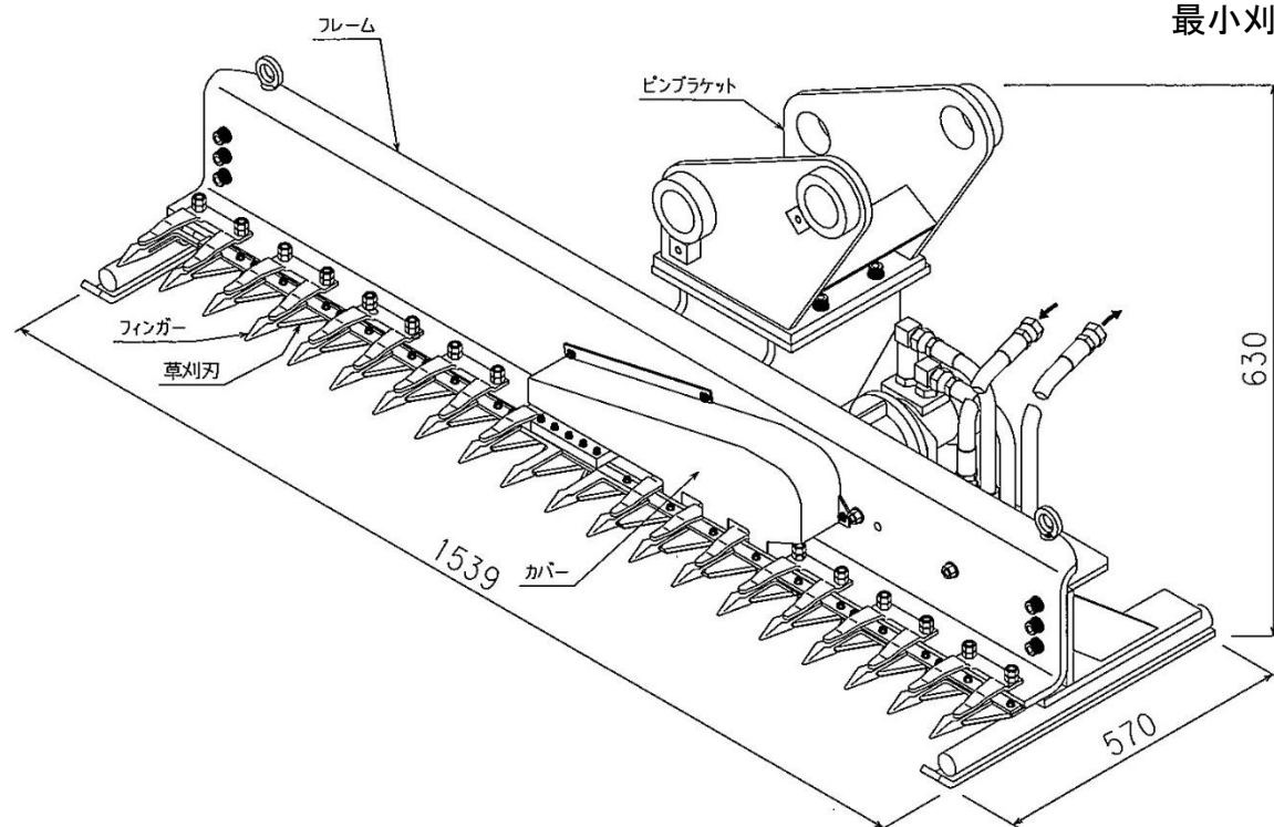
図2. 各部の名称
