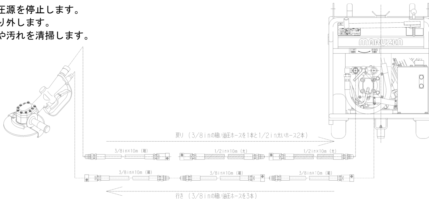
延長ホースの接続例（最長 30m）
