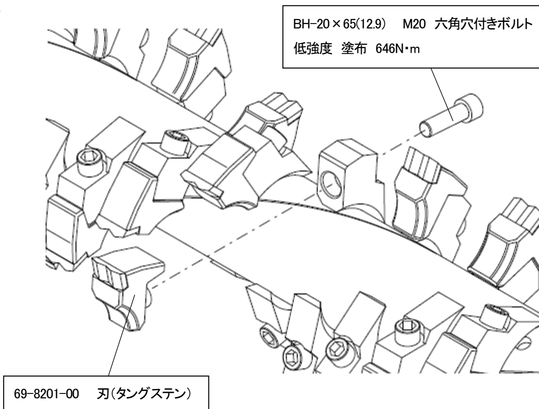
図6. 刃の取り付け方法
