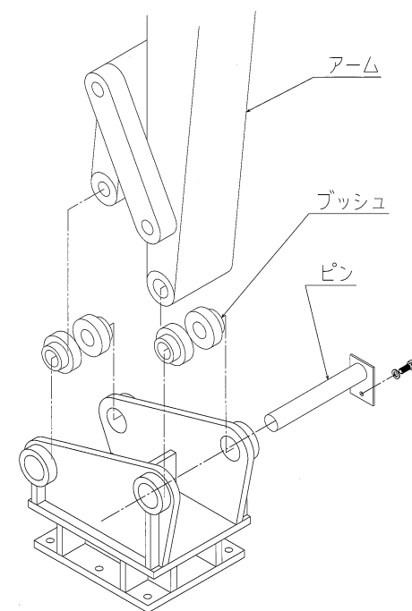
図5. 油圧ショベルへの取り付け方法
