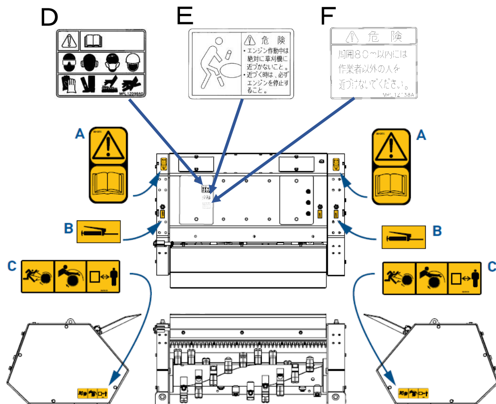
図1. 安全標識の貼り付け位置
