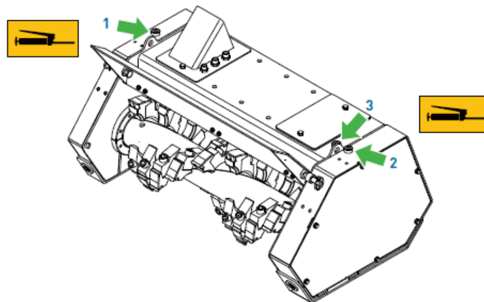
図7. グリス注入位置
