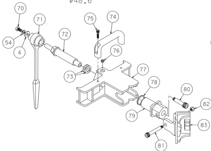
単管クランプ (EH34-48) φ48.6
