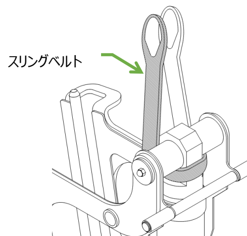
本機の吊り上げ方
