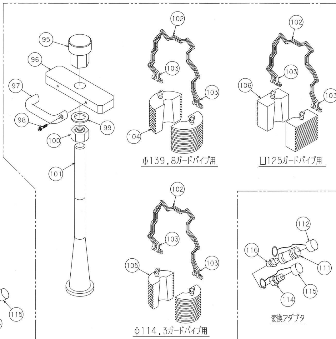
内抜き治具 (EH34-B)
