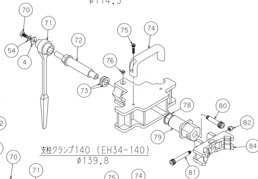
支柱クランプ114 (EH34-114) φ114.3
