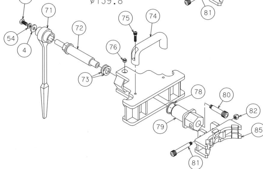
支柱クランプ140 (EH34-140) φ139.8
